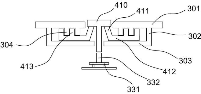
<버튼 스위치 방수구조>
